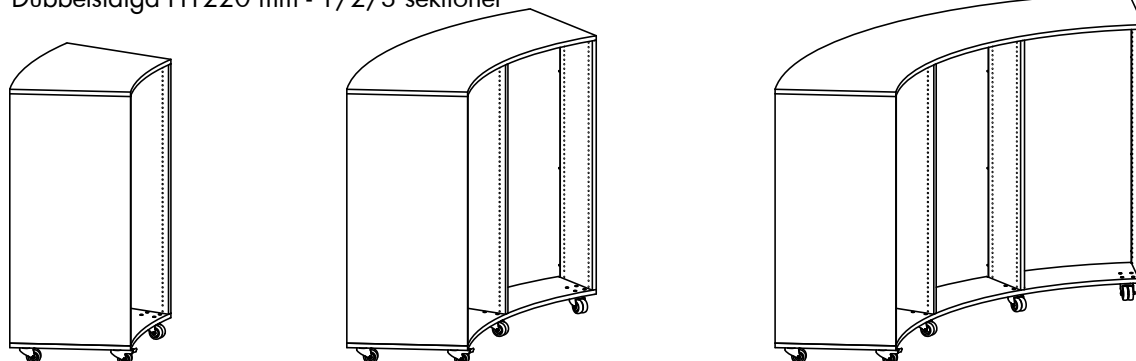
Dubbelsidiga H1520 mm - 1/2/3 sektioner
